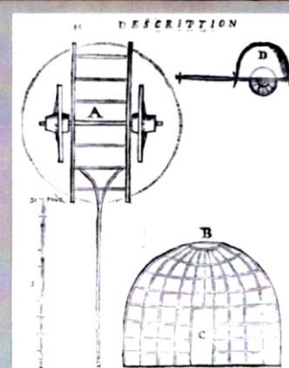
Figure 9.2 Nogay cart-tent, c. 1645 (after Guillaume Le Vasseur, Sieur de Beaucaplan, Description d'Ukraine, qui sont plusieurs Provinces du Royaume de Pologne, Rouen, 1660, p. 30)
